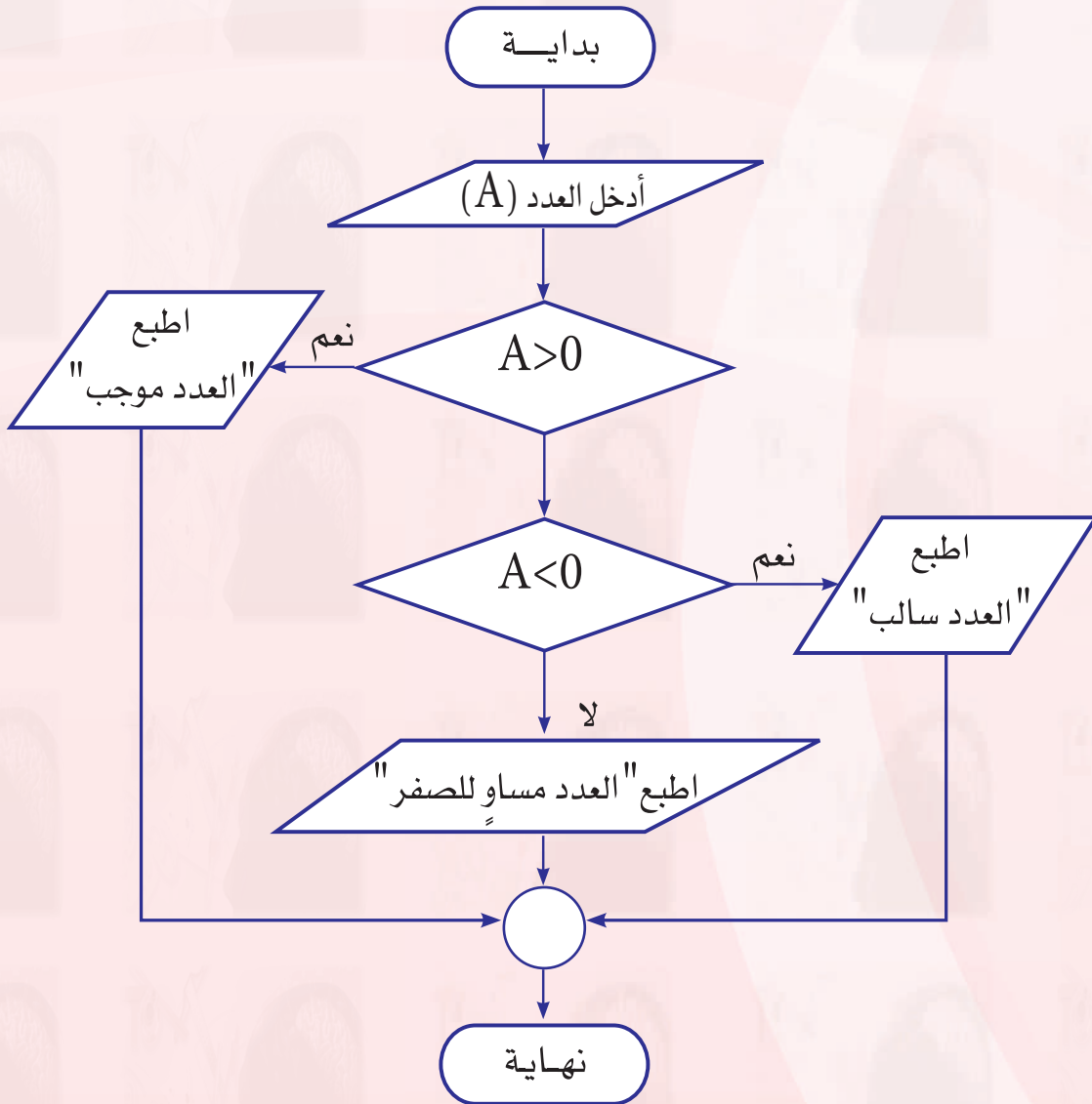
شكل (٦-٣) : مخطط انسياب لتحديد العدد سالب أم موجب
