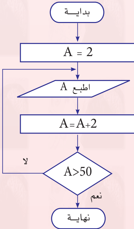
شكل (٦-٥) : مخطط انسياب طباعة الأعداد الزوجية
