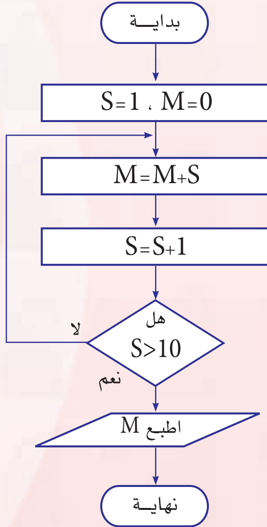
شكل (٢-٦) : مخطط انسياب مجموع الأعداد من (1) إلى (10)
