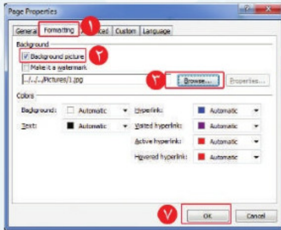
شكل (١١-٢-٥): تغيير الخلفية كصورة
